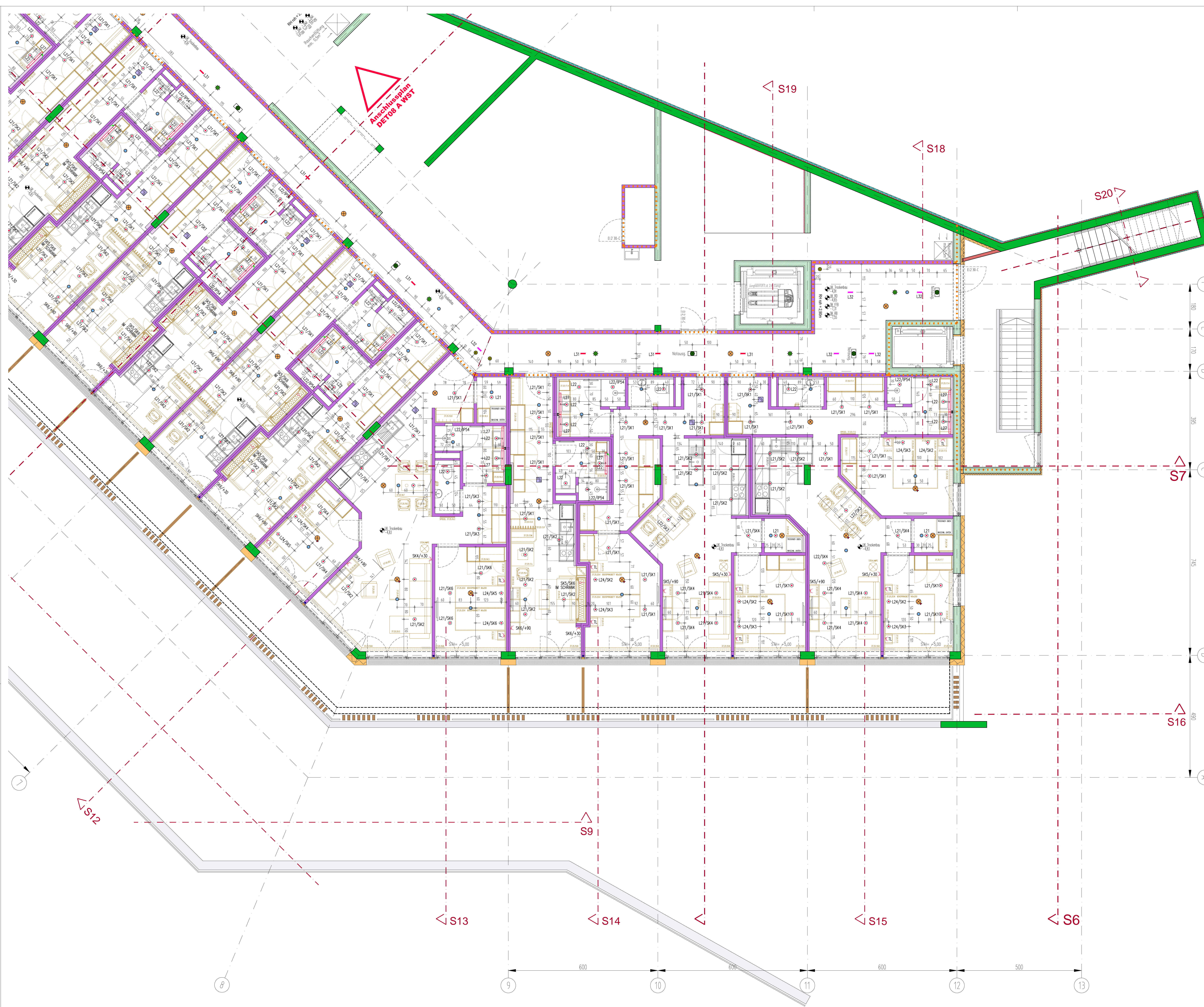
DECKENSPIEGEL UG2 OST - 1:50
